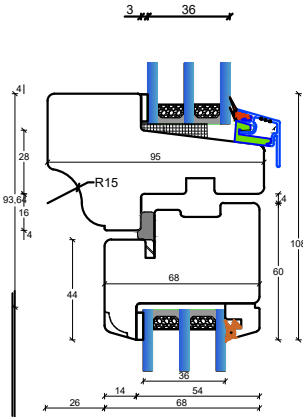
L5: Lodpost, fast/åbenbar vandret med R15 almue
