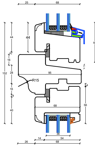
L5: Lodpost, fast/åbenbar vandret med R15 almue
