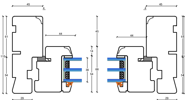
V3: Sidekarmer åbenbare eller faste partier med ramme
