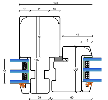
V5: Topkarm åbenbare eller faste partier med ramme
