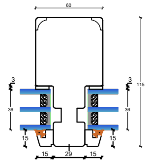
L2: Lodpost, fast/fast lodret
