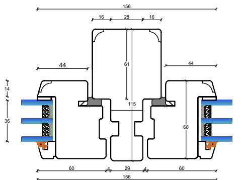
L4: Lodpost, fast/åbenbar lodret
