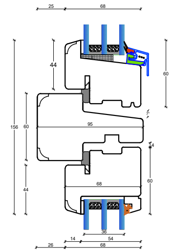
L5: Lodpost, fast/åbenbar vandret
