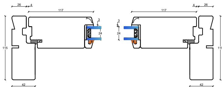
D2: Topkarme døre, udadgående
