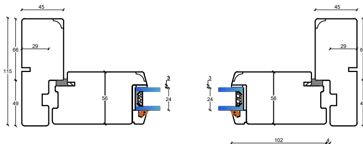
D1: Sidekarme døre, udadgående
