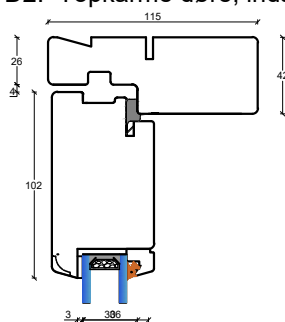
D2: Topkarme døre, indadgående
