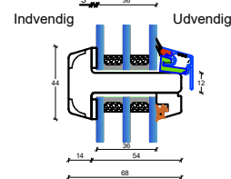
45 mm. gennemgående sprosse Modern
