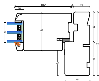
D2: Topkarme døre, indadgående
