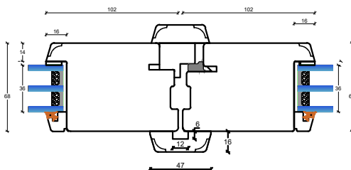
L1: Lodpost lodret
