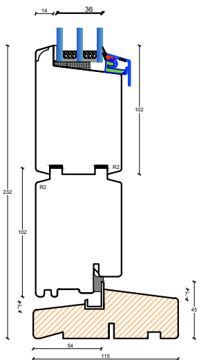
L2: Lodpost vandret
