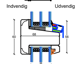
56 mm. gennemgående sprosse Modern
