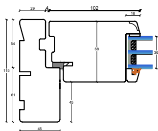
D2: Topkarme døre, udadgående
