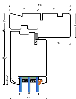
D2: Topkarme døre, indadgående
