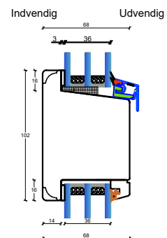
105 mm. gennemgående sprosse Modern
