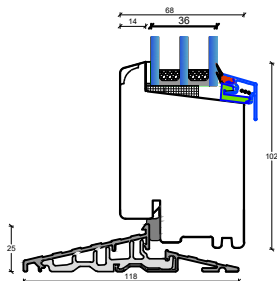
D3: Dørtrin udadgående dør (kan leveres med dobbelt spændestykke)
