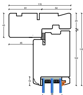
D2: Topkarme døre, udadgående
