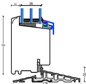
D3: Dørtrin indadgående dør (kan leveres med dobbelt spændestykke)
