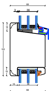
L2: Lodpost vandret
