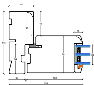
D1: Sidekarme døre, udadgående
